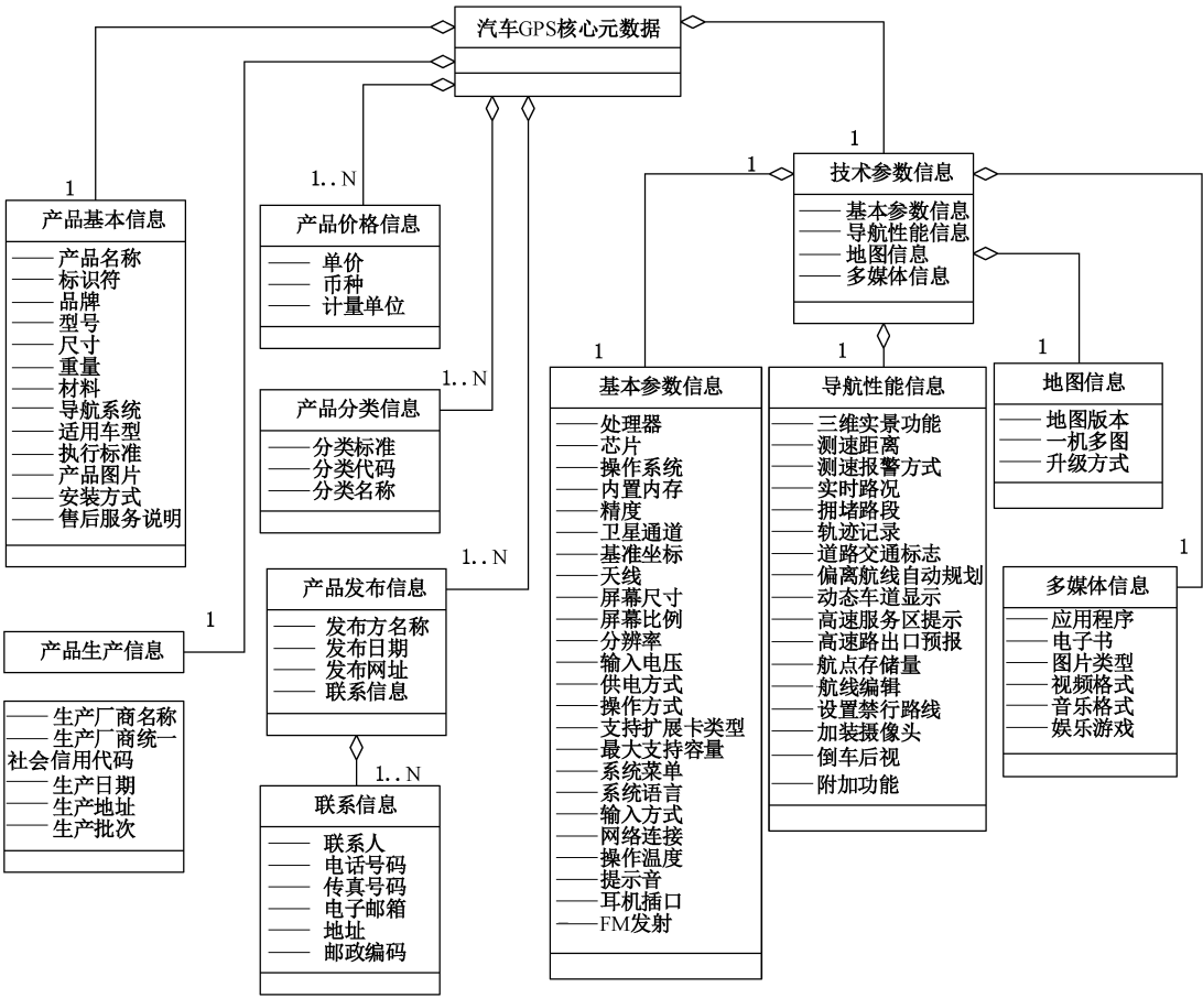
图 1 车载导航终端核心元数据统一建模语言描述
